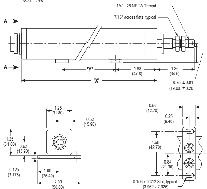
VIEW A-A
